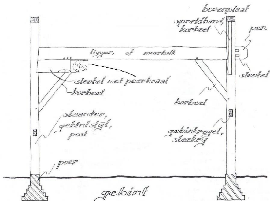
Gebint opzet van een houten huis, bouwmethode 15 e en 16 e eeuw
