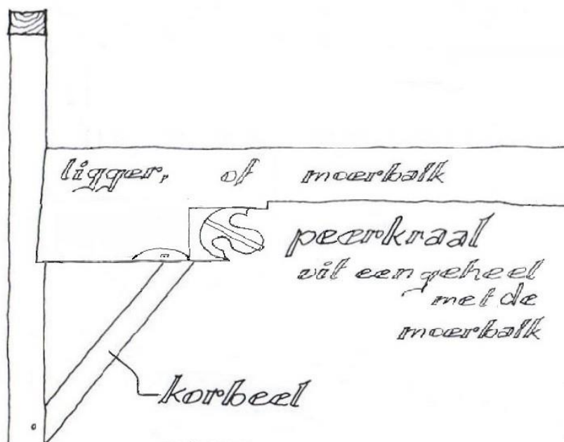
Schets van de peerkraal zoals die aangetroffen is in Langestraat 131. Het unieke van deze vondst is dat de peerkraal uit de moerbalk is gebeiteld en één stuk vormen zonder sleutelstuk.
